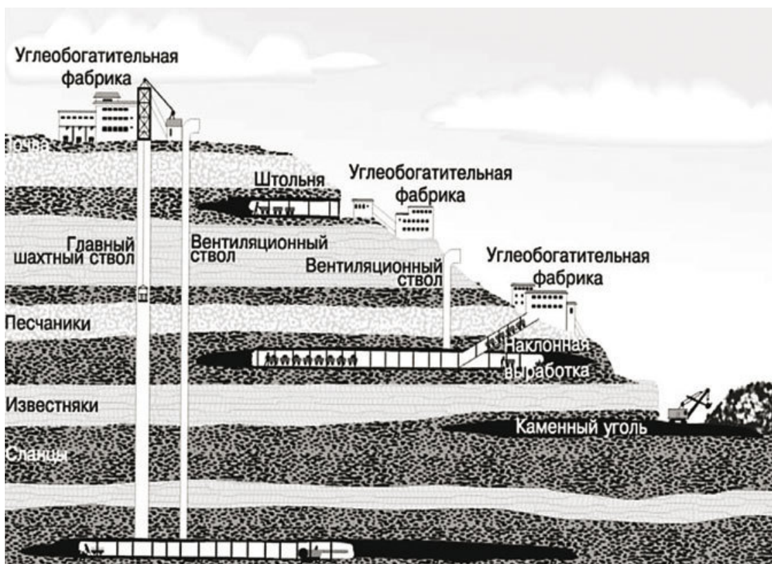
Схема залегания и разработки угольных пластов
