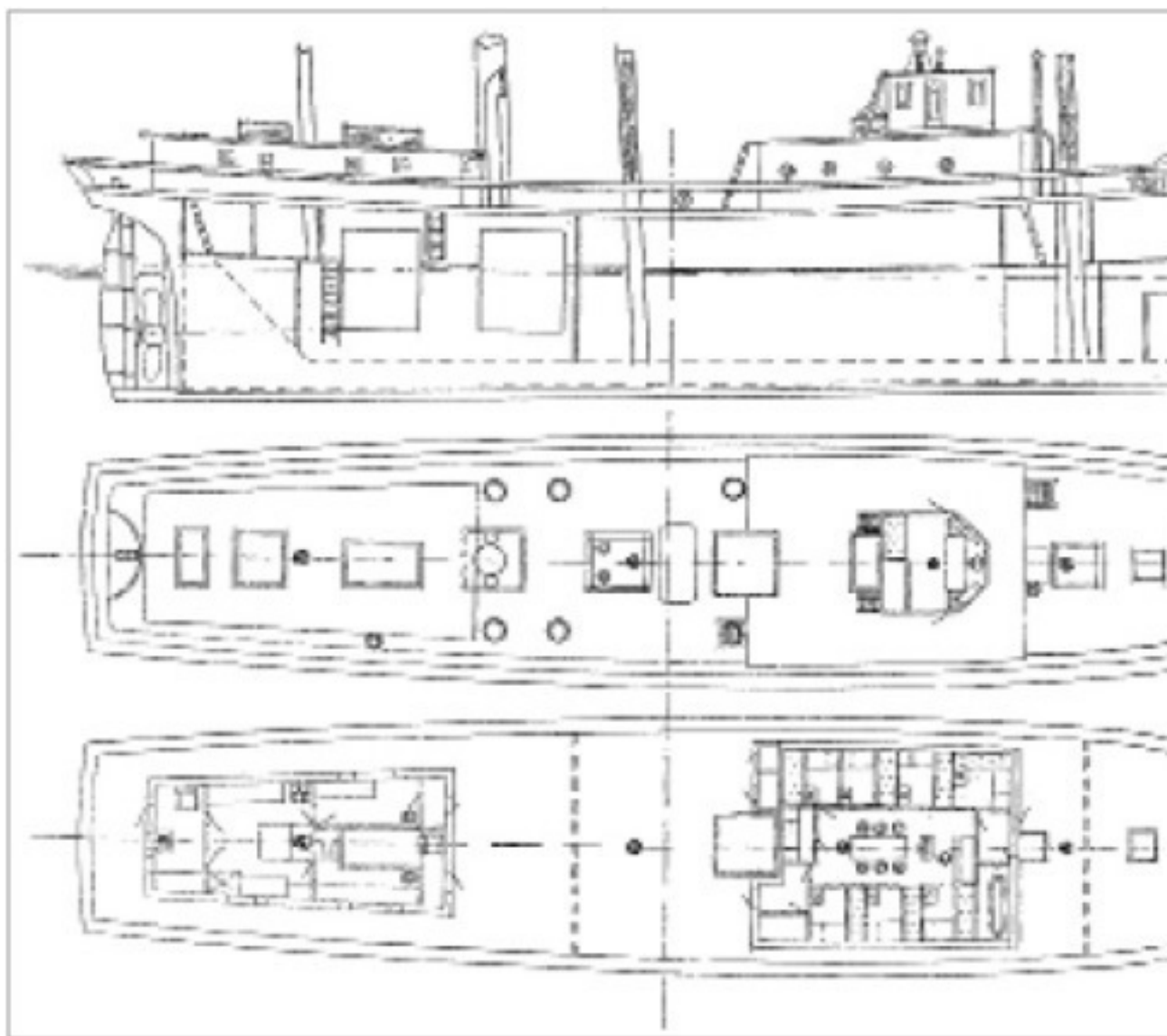
Схема общего расположения яхты «Заря»
