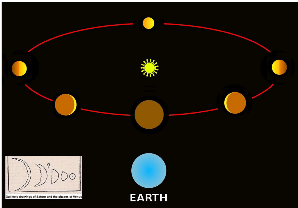
Фазы Венеры, зарисованные Галилеем и изображенные схематически.
