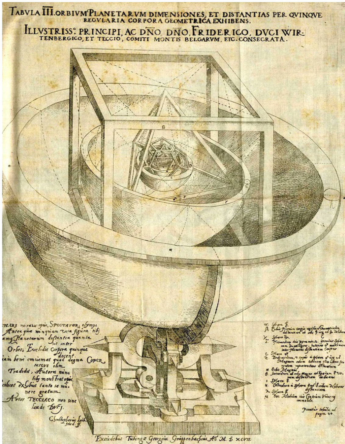
Гелиоцентрический кубок шести планет Кеплера.
