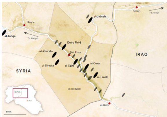
Карта нефте-и газовых месторождений в провинции Дейр эз-Зор
