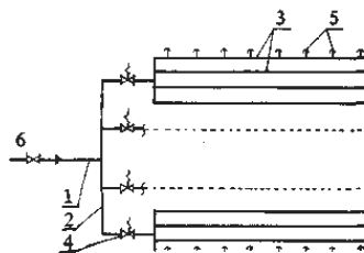
Рис. 9. Трубопроводы: – магистральный; 2 – распределительный; 3 – подводный пластмассовый; 4 – магнитный клапан; 5 – форсунка; 6 – вода (питательный раствор).
