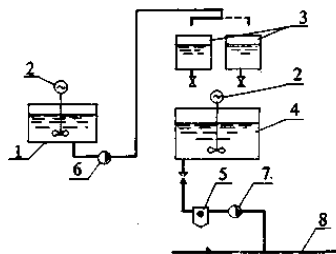
Рис. 10. Растворный узел:
