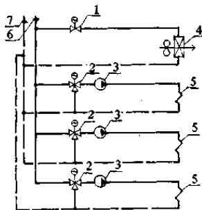
Рис. 7. Принципиальная схема отопления:
