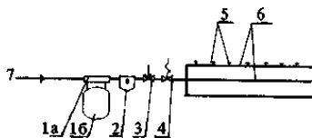
Рис. 13. Система с дозатором:
