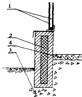
Рис. 8. Поперечное сечение:
