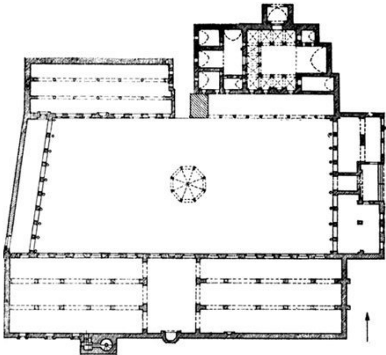
Диярбакыр. Улу-джами. План
