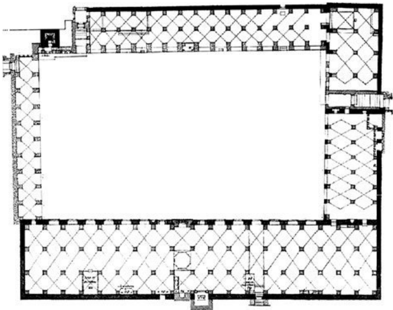
Алеппо. Джами аль-Кабир. План
