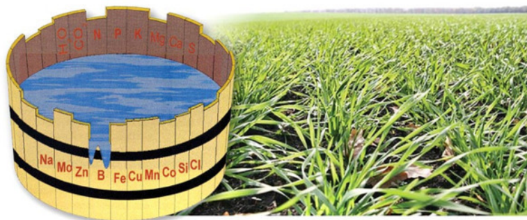
Рис. 6 – «Бочка Либиха»
