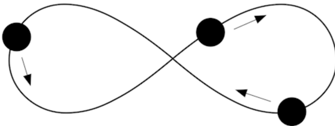
Орбита для трех тел в форме восьмерки
