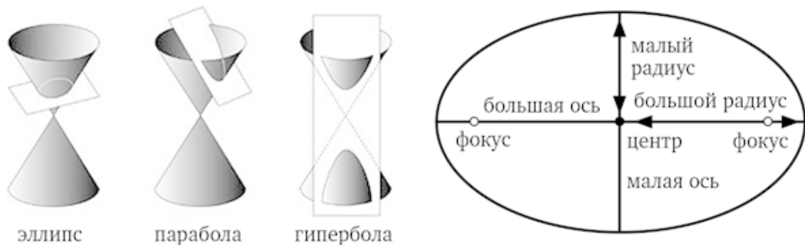
Слева: конические сечения.
