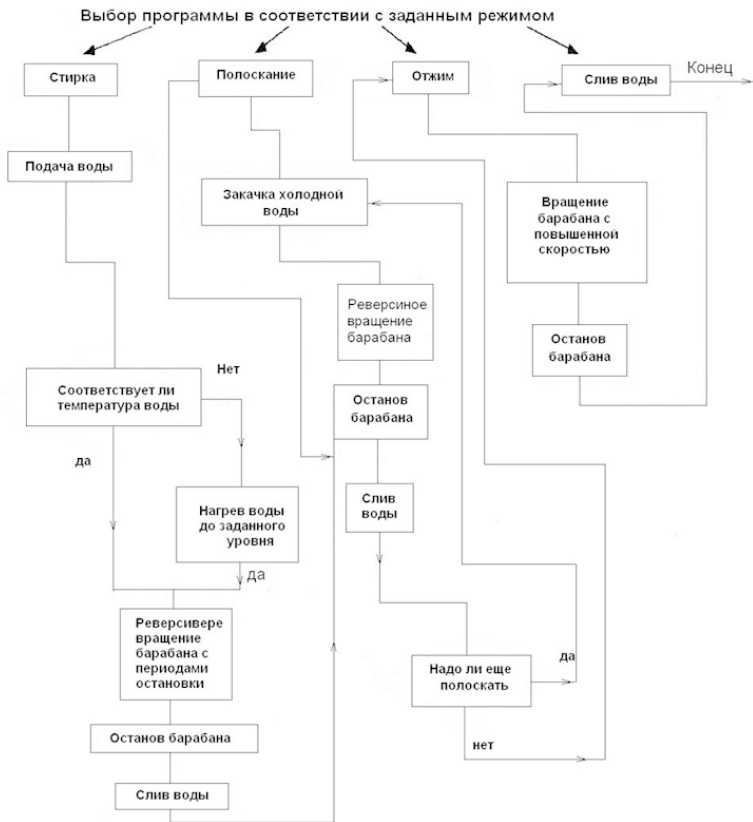
Рисунок 1.7 – Блок-схема работы стиральной машины СМА-4ФБ «Вятка-автомат-12»
