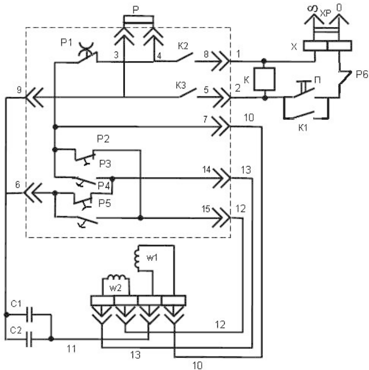
Рисунок 1.4 – Стиральная машина типа СМР
