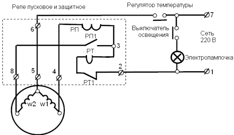
Рисунок 2.2 – Электрическая схема холодильника.
