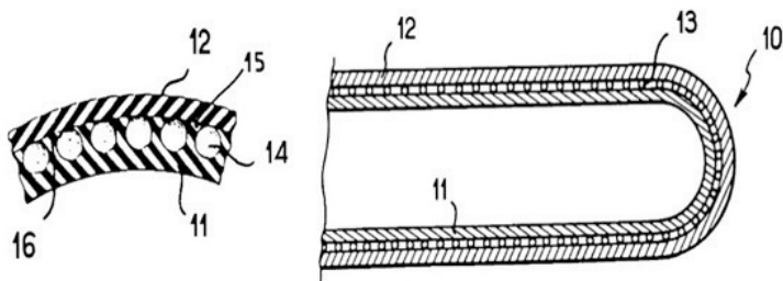
Рис. 3.4. Хирургическая перчатка. Патент США 5 024 852
