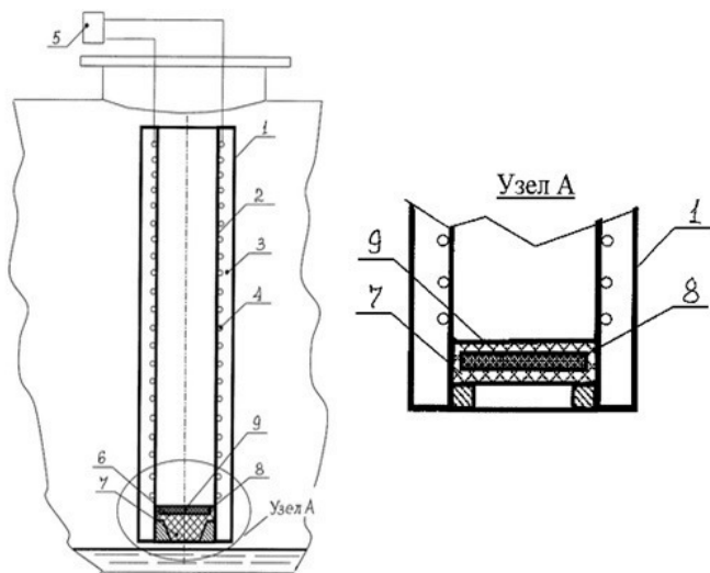
Рис. 4.7. Датчик
