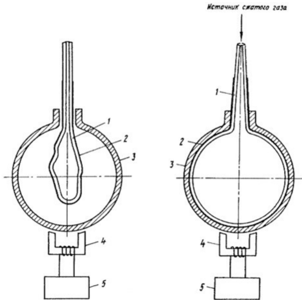
Рис. 4.8. Измеритель толщины. А. с. 792 080
