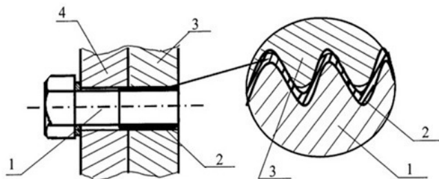
Рис. 4.3. Болтовое соединение. Патент РФ 2 256 108 1 – болт; 2 – слой нитинола; 3, 4 – соединяемые детали.
