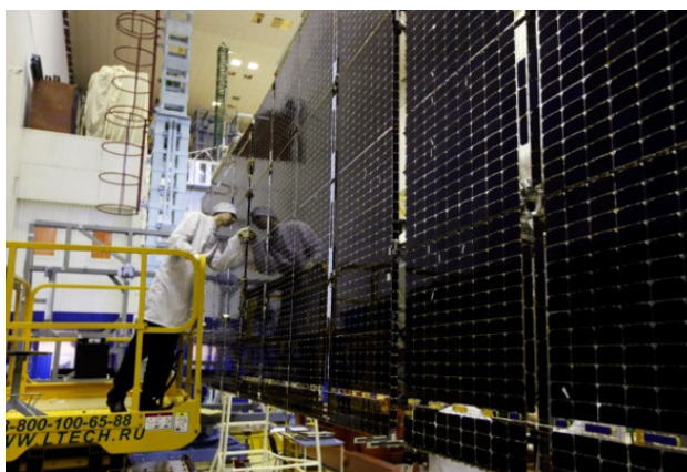
Тестирование солнечных батарей КА «Amos-5»
