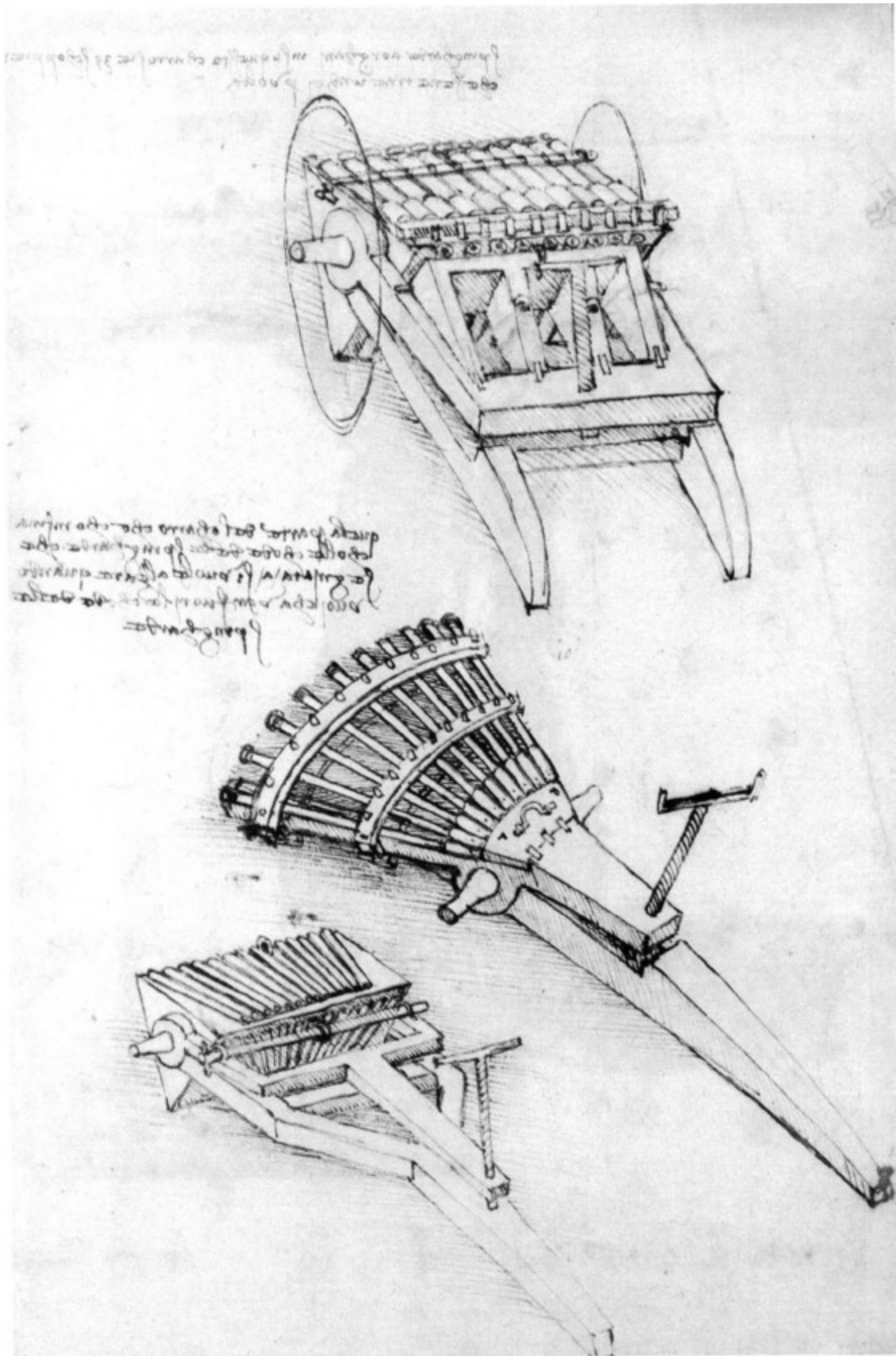
Леонардо да Винчи. 33-ствольная пушка
