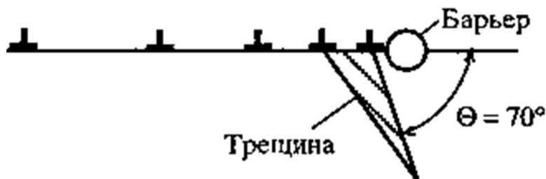
Рис. 3. Схема зарождения трещины у вершины дислокационного скопления [3]
