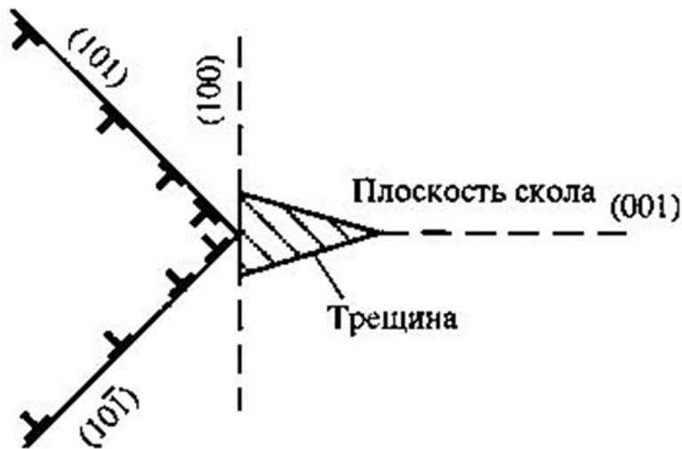
Рис. 4. Схема зарождения трещины в ОЦК металлах [3]
