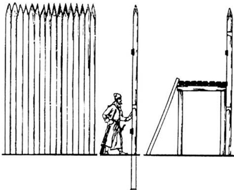
Рис. 6. Устройство тына
