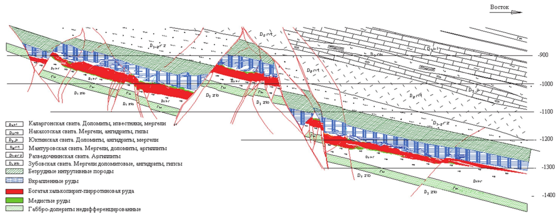
Рис. 1. Разрез по Харлаелаксской I рудной залежи
