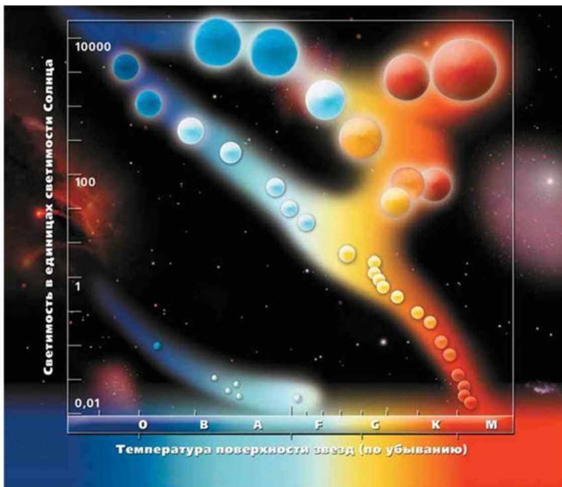
Рис. 1.1. «Жизненный путь» звезд – по мере старения звезда обнаруживается в различных точках изображенной на рисунке диаграммы Гершпунга – Рассела, чаще всего движение идет по «главной последовательности» – линии точек, идущей из верхнего левого угла диаграммы в нижний правый.
