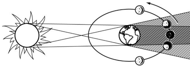
Схема лунного затмения
