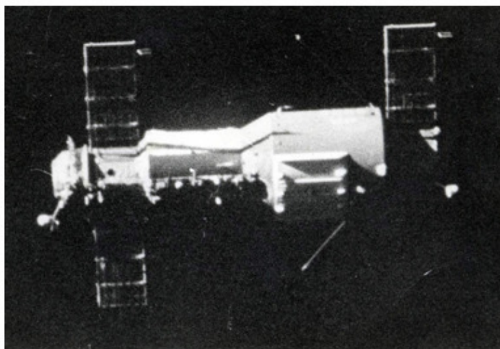
Космическая станция «Салют-1». Уникальный снимок с космического корабля «Союз-11».
