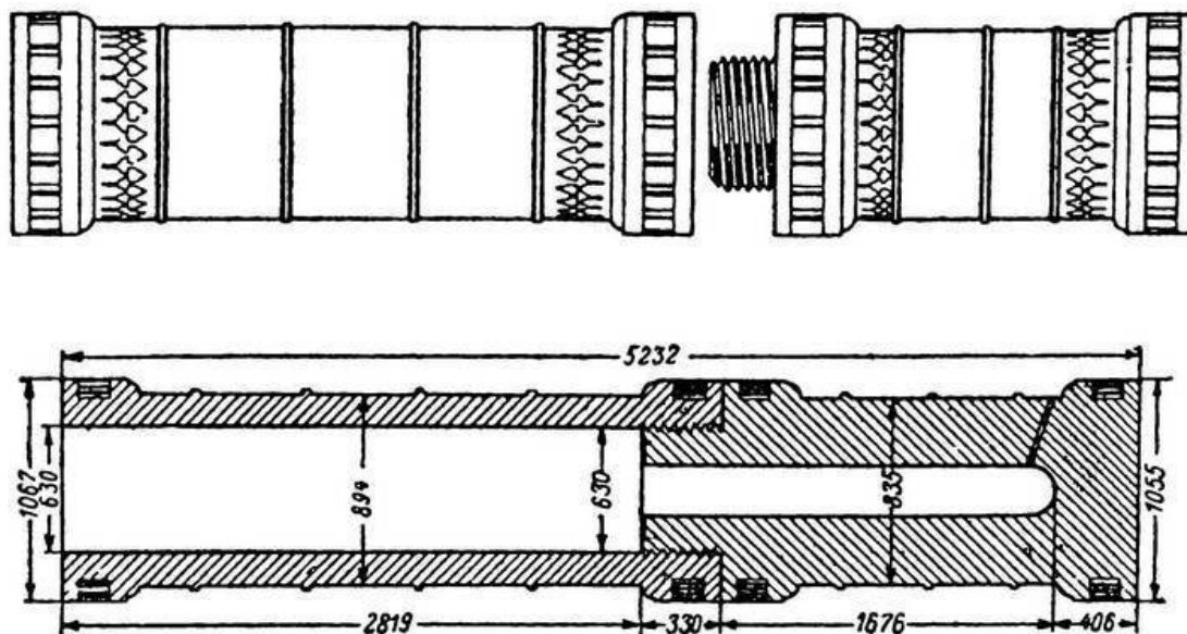
25-дюймовое (63,5-см) бронзовое турецкое орудие
