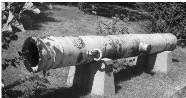
Стенобитная 260-мм пушка с длиной ствола 3570 мм, отлитая в 928 г. мастером Хайреддином бин Абдуллой. Стамбул. Военный музей. (Фото А. Широкограда)
