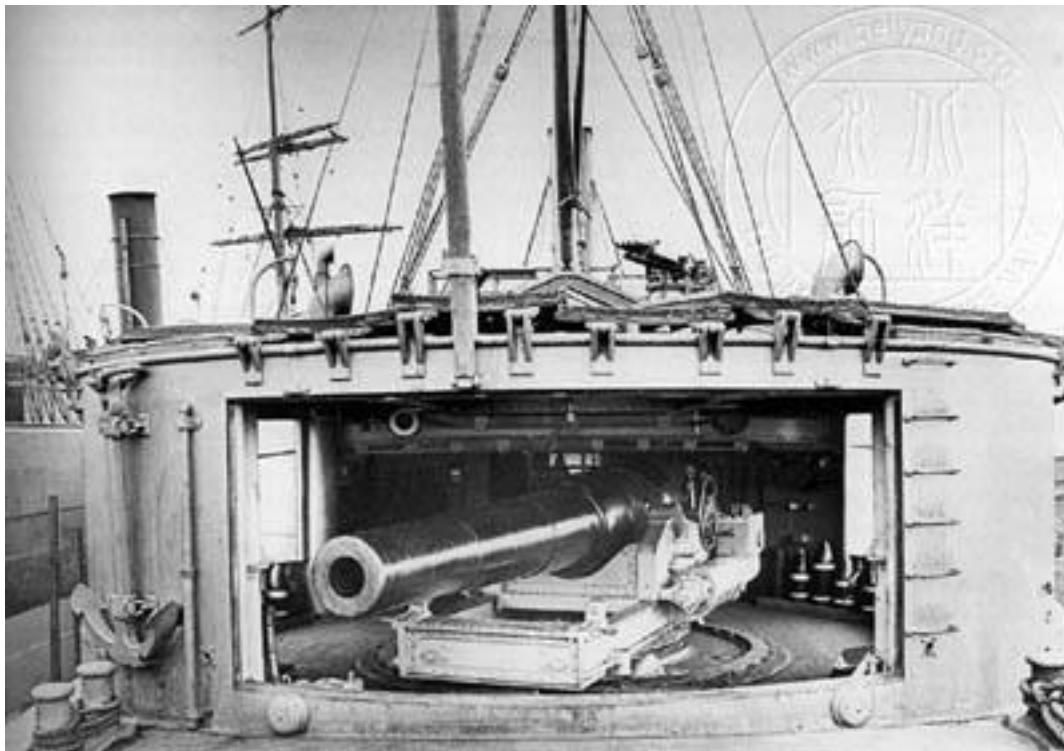
Фото 20 – 10-дюймовое орудие Армстронга.
