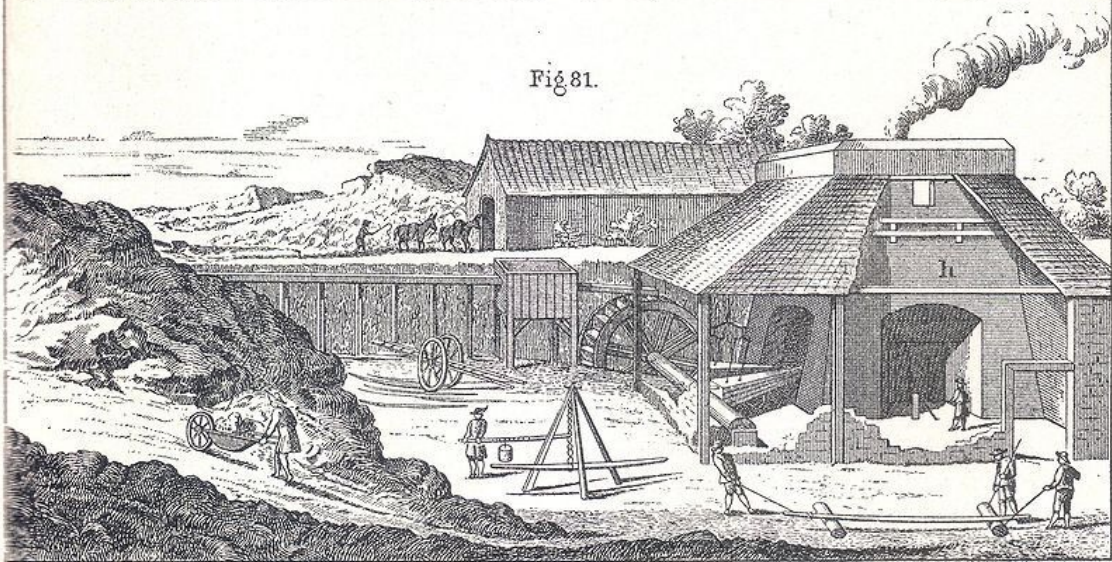
Disposition d'un haut-fourneau au commencement du xviii e siècle.
