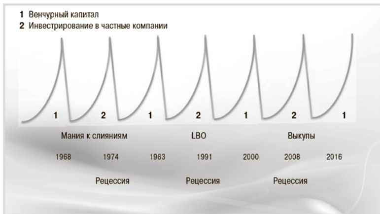
Рис. 1.1. Волна Дрейпера
