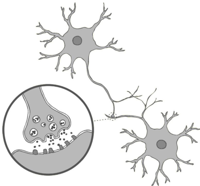
Нейроны и их связи
