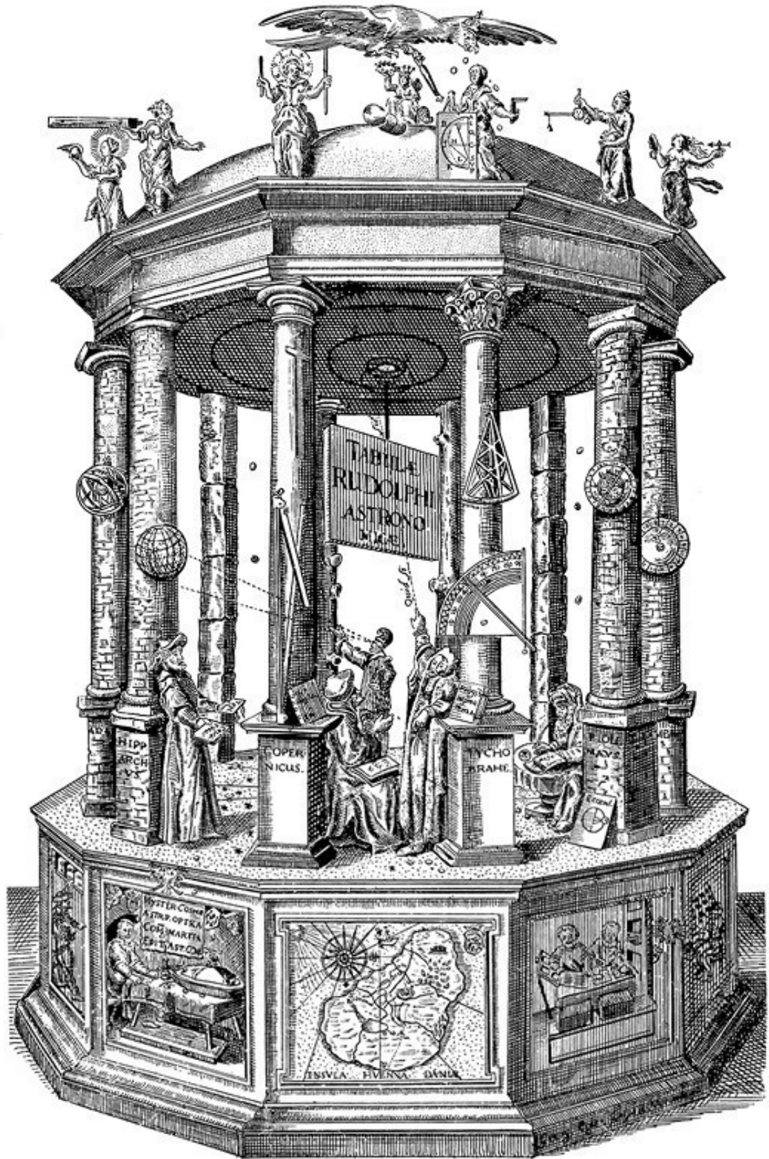
Фронтиспис к «Рудольфовым таблицам» (1627 г.) Иоганна Кеплера, символизирующий историю астрономии. На нем представлен храм Урании, где расположились Гиппарх, Коперник, Тихо Браге и Птолемей с различными инструментами. На карте (внизу по центру) изображен остров Вен, где работал Тихо Браге. Обратите внимание на телескоп Кеплера (вверху
