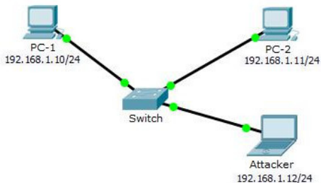
Рисунок 38 – Схема лабораторного стенда
