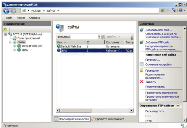
Рисунок 19 – Процесс настройки сайта
