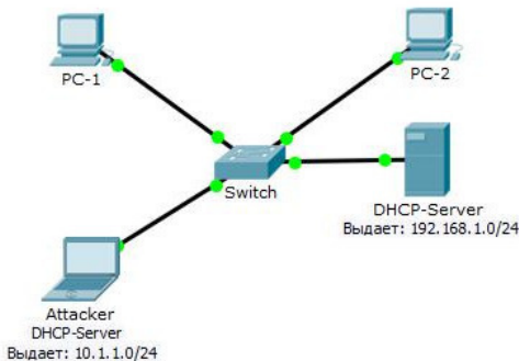
Рисунок 46 – Схема лабораторного стенда
