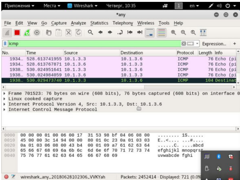
Рисунок 39 – Перехват пакетов
