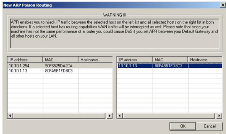
Рисунок 43 – Вкладка ARP
