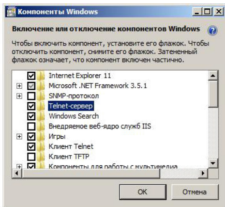
Рисунок 31 – Выбор Telnet-сервера
