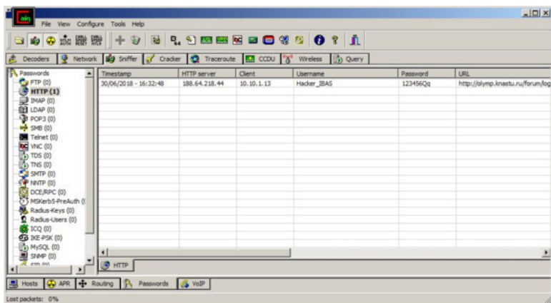
Рисунок 45 – Получение логина и пароля жертвы
