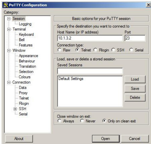
Рисунок 33 – Подключение через протокол Telnet
