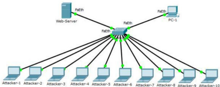
Рисунок 56 – Схема лабораторного стенда
