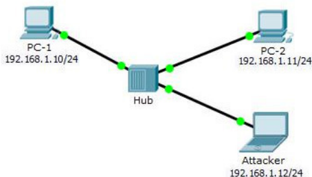
Рисунок 1 – Лабораторный стенд для проверки уязвимости
