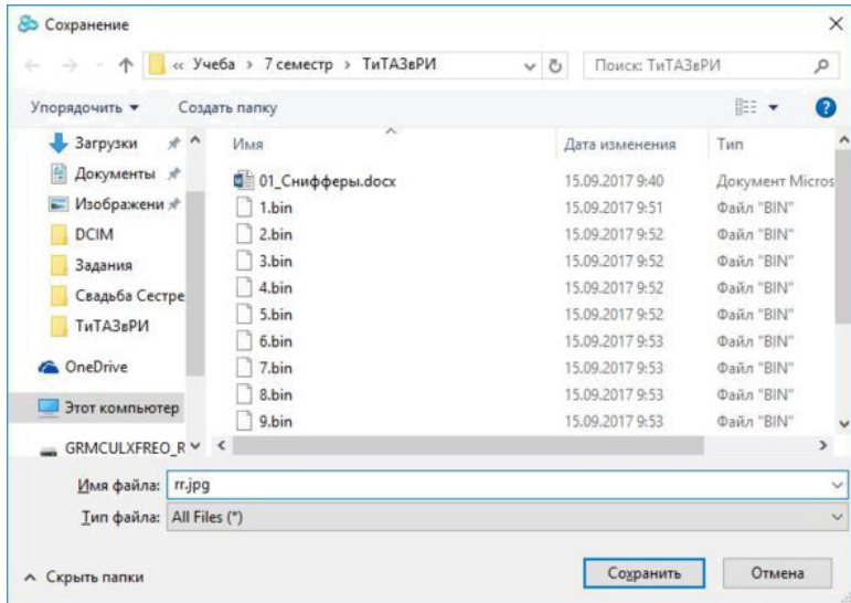
Рисунок 14 – Восстановленные данные
