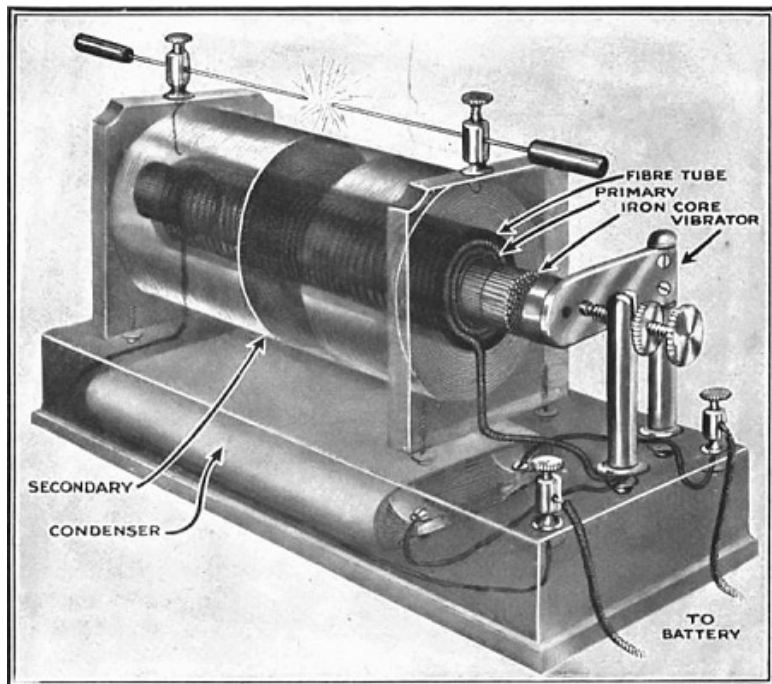
Индукционная катушка Румкорфа.
