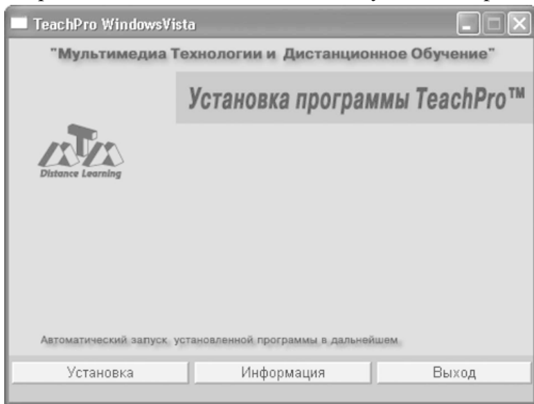
Рис. 01. Диалоговое окно начала установки программы
