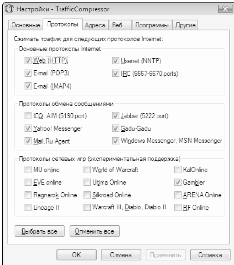
Рис. 1.6. Вкладка Протоколы
