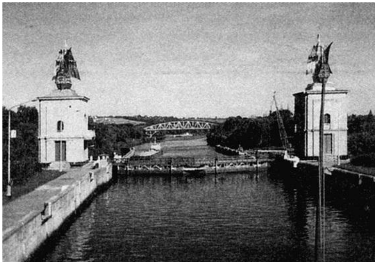
Один из шлюзов канала им. Москвы
