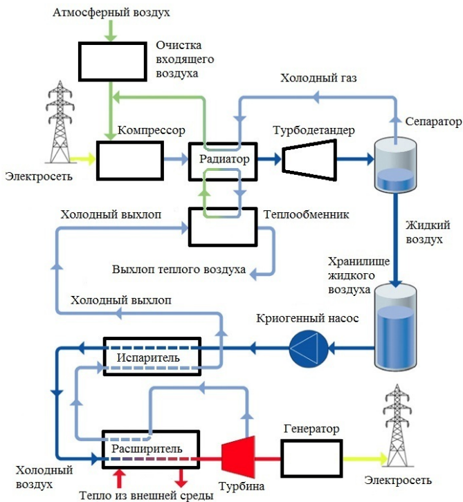
Рис.3.5. Схема основного оборудования криогенной электростанции
