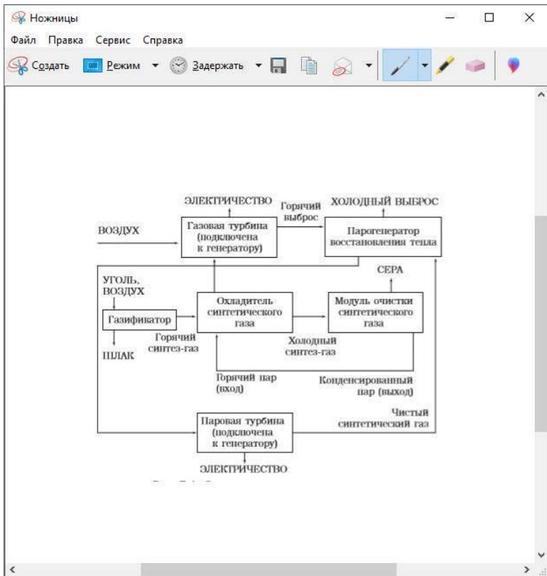
Рис.3.1. Схема станции интегрированного газификационного комбинированного цикла
