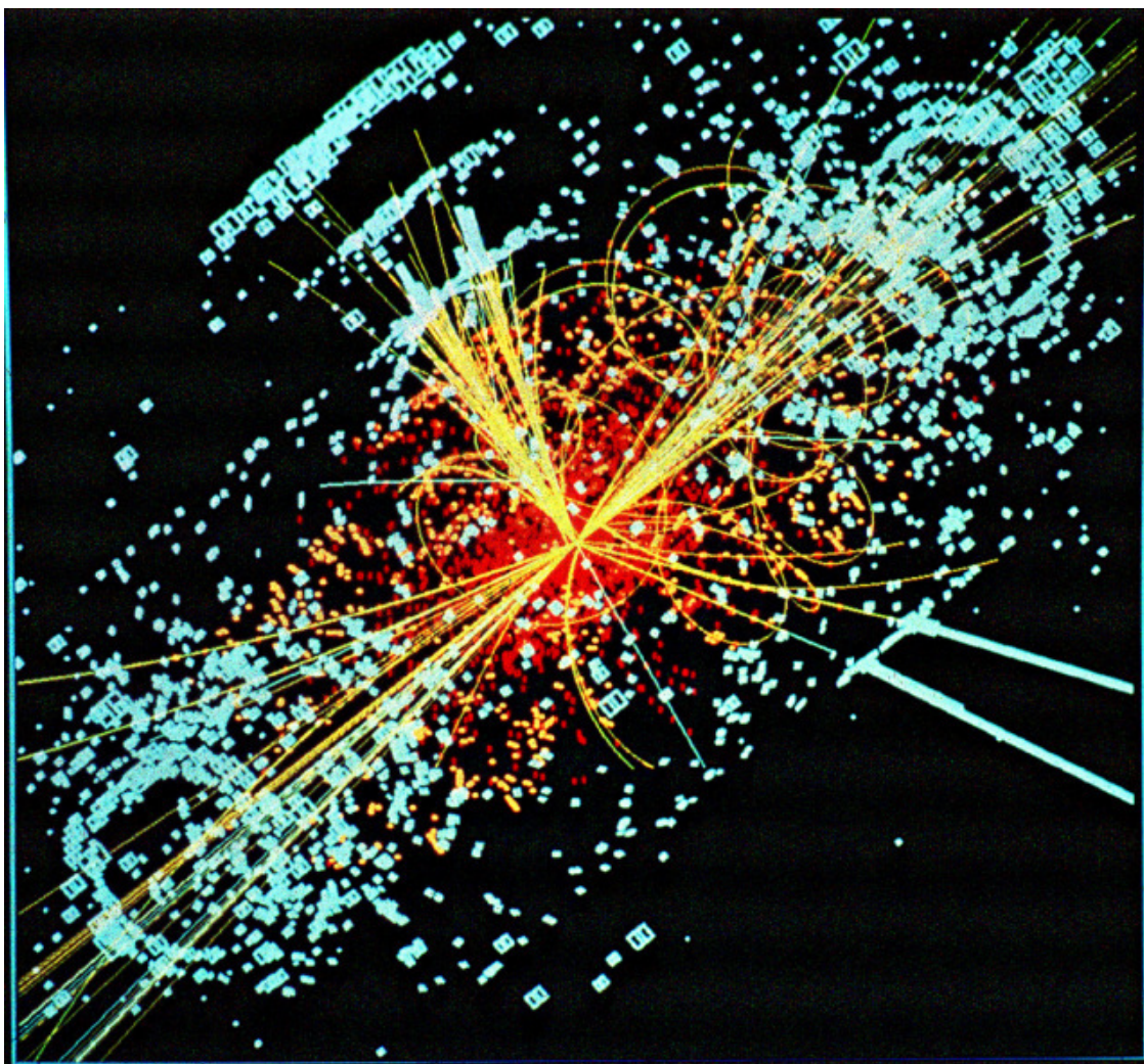
Рисунок 6: Анализ столкновения двух протонов в ЦЕРНе
