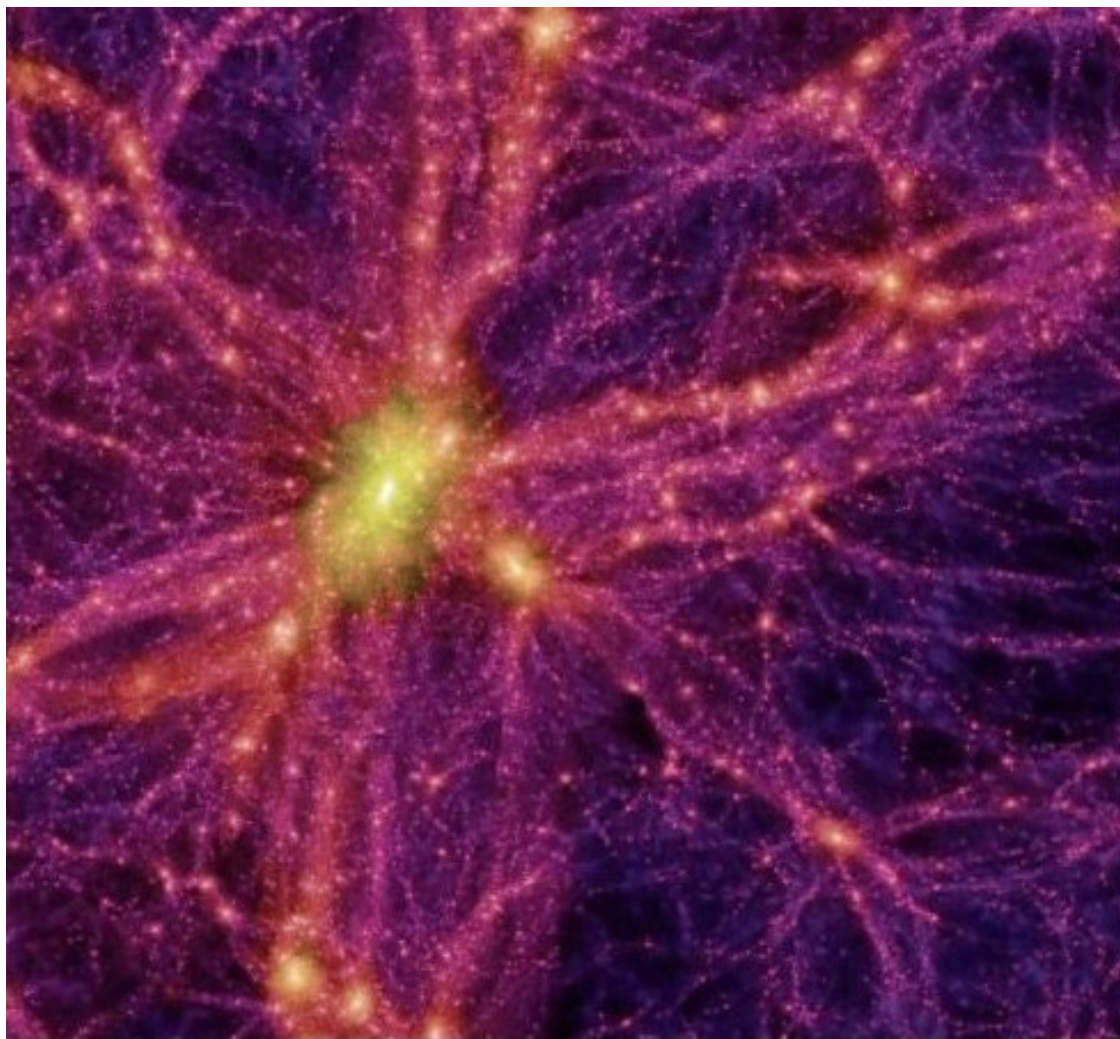
Рисунок 10: Здесь показано выравнивание квазаров на модели крупномасштабной структуры вселенной (European Southern Observatory). Синим цветом моделируются распространения тёмной материи среди туманностей, квазаров (очень ярких галактик), скоплений и сверхскоплений. Пространства между венами обозначают космические пустоты или супервойды.
