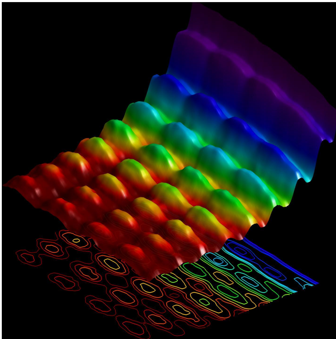
Рисунок 3: Фотография света как частиц в волнах (EPFL)
