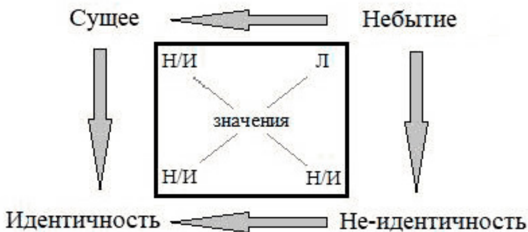
Рисунок 15: Логический квадрат
