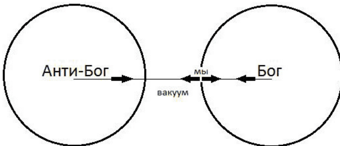
Рисунок 16: Упрощённая визуализация динамики Источников (уровня 15) Модели
