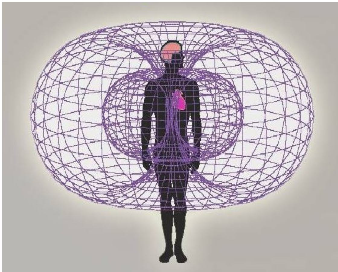
Рисунок 2: Иллюстрация физического био-электромагнитного поля, порождённого нашим сердцем (HeartMath). Там же имеются более свежие иллюстрации, которые показывают биополе сердца в отношении к телесному биополю.
