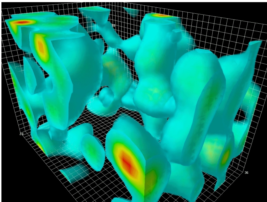
Рисунок 5: Содержимое пространства внутри атома
