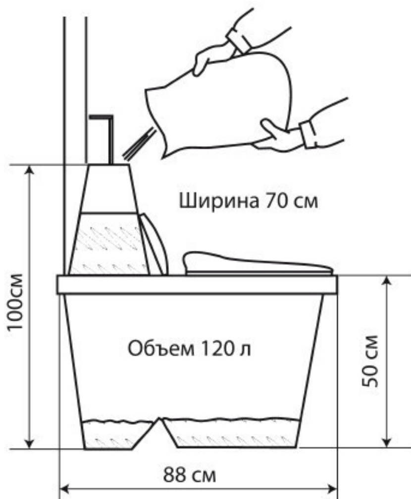
Рисунок 3. Торфяной биотуалет (разрез)
