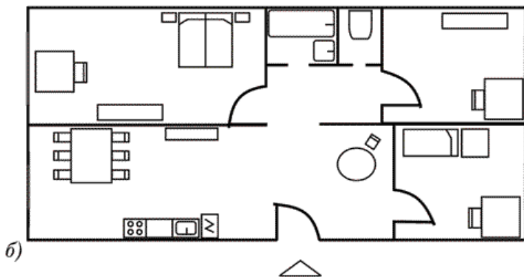
Рис. 2. Предполагаемые варианты перепланировки: а) вариант 1; б) вариант 2
