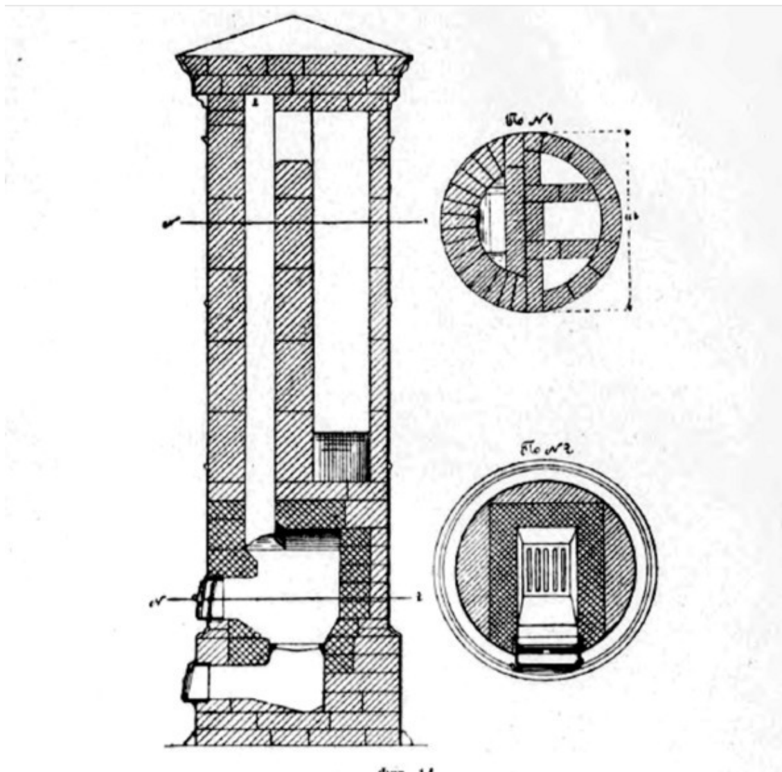
В. Пересвет-Солтан. «Проектирование комнатных печей» 1911 г.
