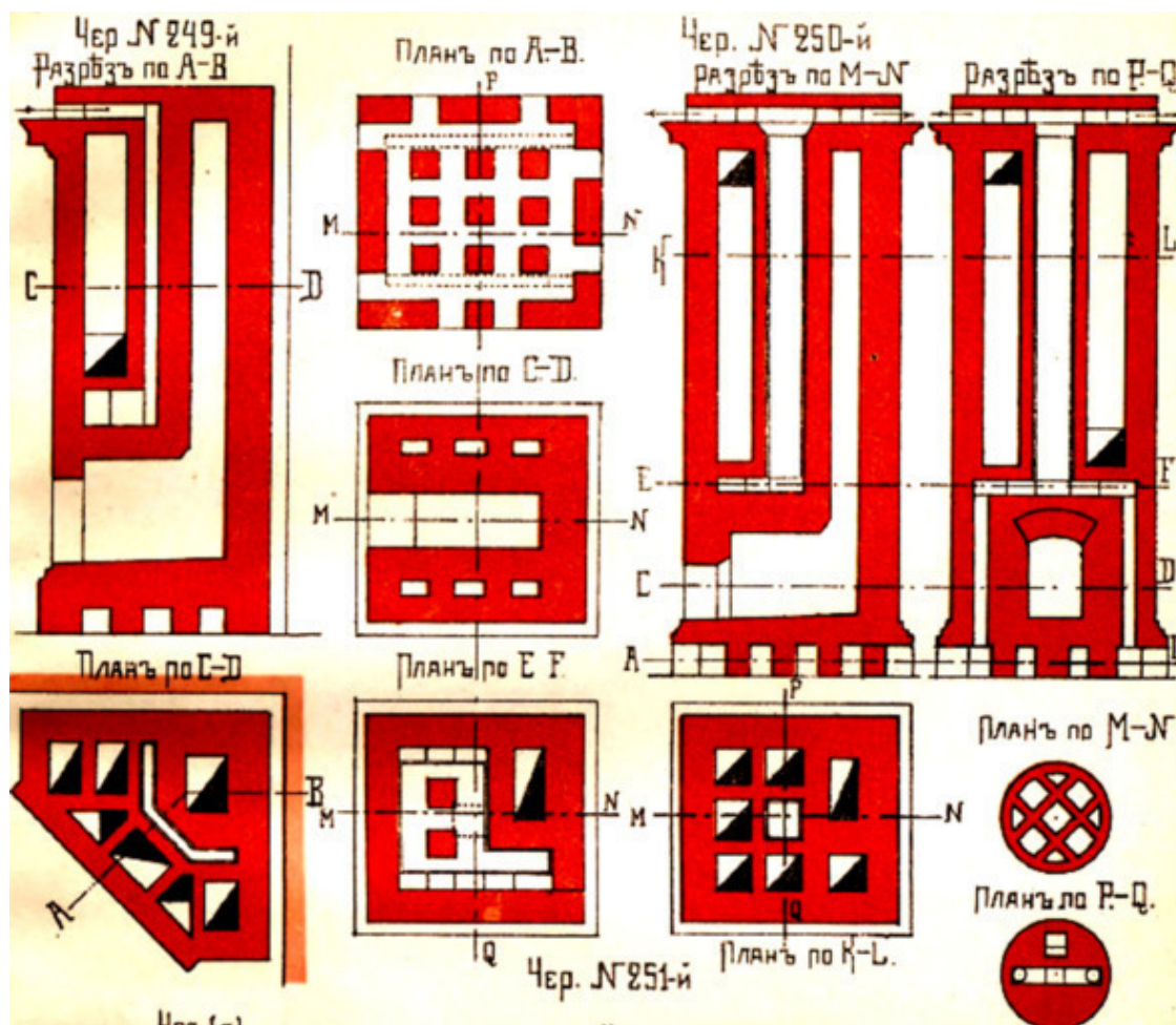
«Кирпичные комнатные печи большой теплоемкости» И. Цыганенко 1913 г.
