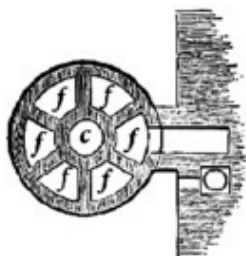
Печь Утермарка (чертёж 1845 г.): а – топливник, б – чугунная плита перекрывающая топливник, с – конвекционный канал, d – отверстия для выпуска воздуха, e – отверстия для впуска воздуха в конвекционный канал, f – ходы, g – вьюшка.
