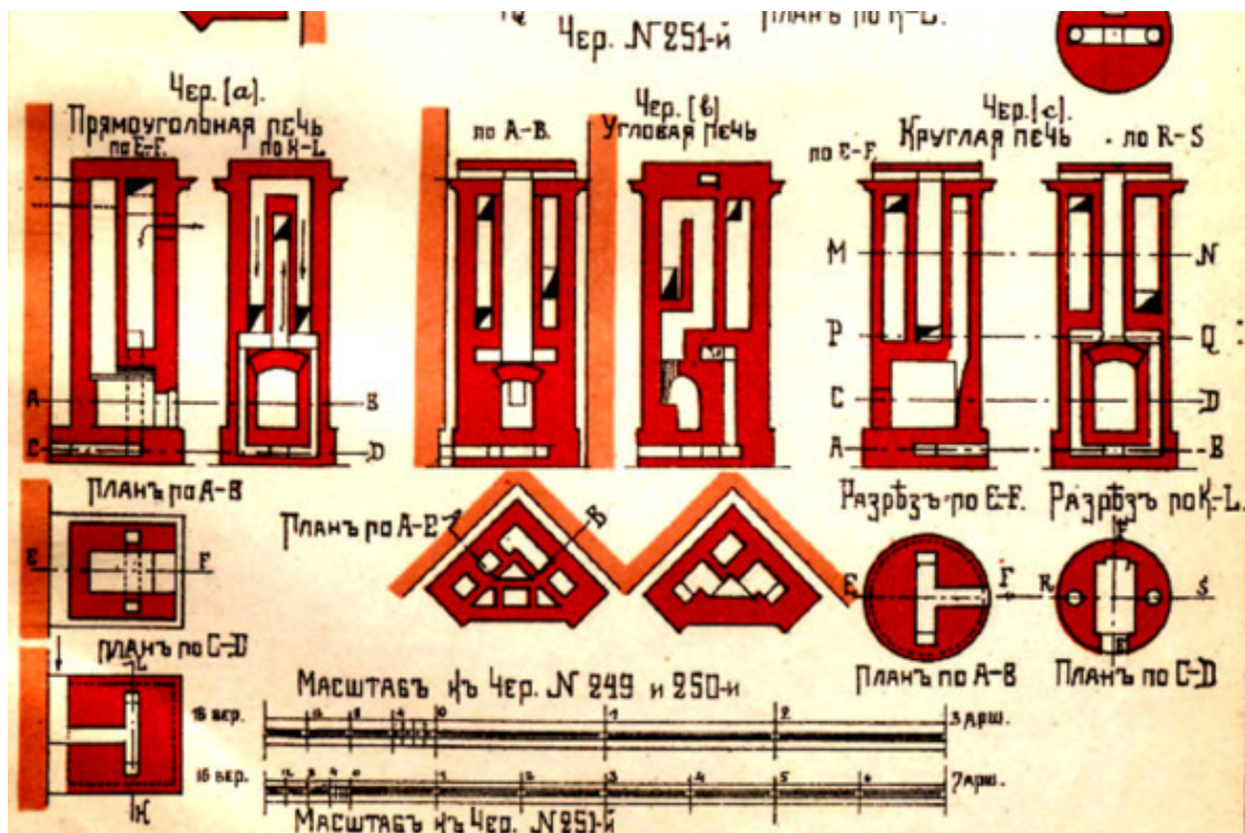
«Кирпичные комнатные печи большой теплоемкости» И. Цыганенко 1913 г.
