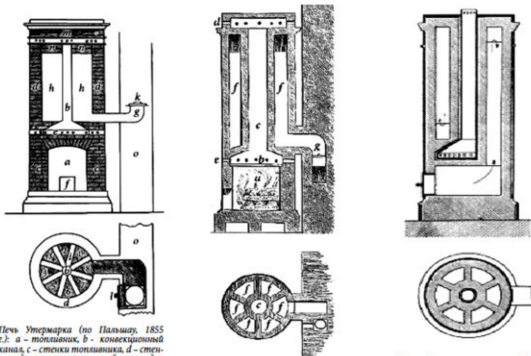
Печь Утермарка с выводом для воздуха сверху. Словарь Брокгауза и Ефрона приводит этот рисунок в качестве изображения оригинальной печи Утермарка.
