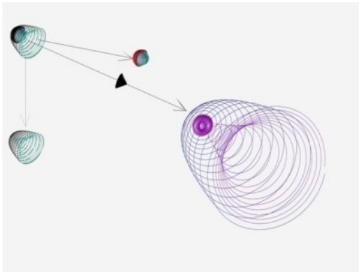
Фото 10. Распад нейтрона
