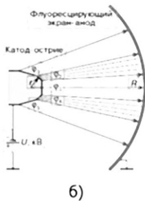
Фото 26. Полевой эмиссионный электронный микроскоп:
