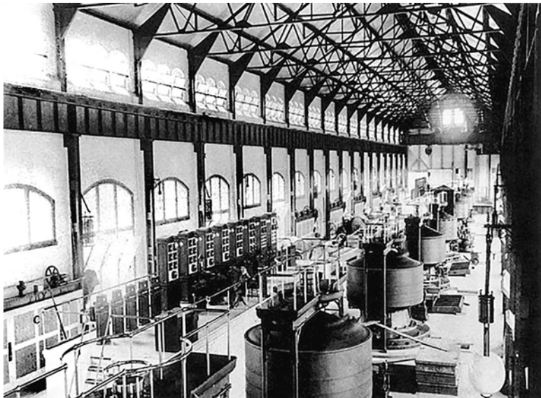
Фото 5. Машинный зал Ниагарской ГЭС, ориентировочно 1897 г.
