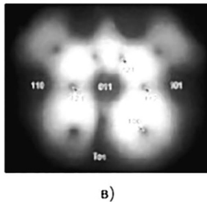
Фото 26. Полевой эмиссионный электронный микроскоп:
