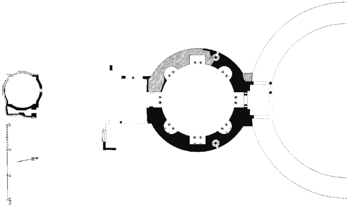
Амастриан. План
