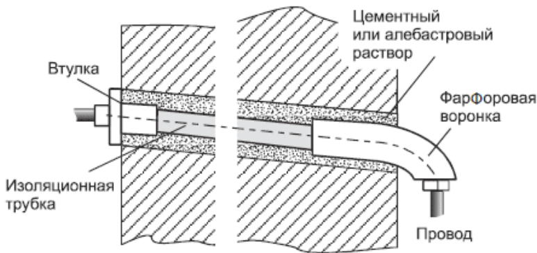
Рис. 1.13. Проход провода ввода через стену
