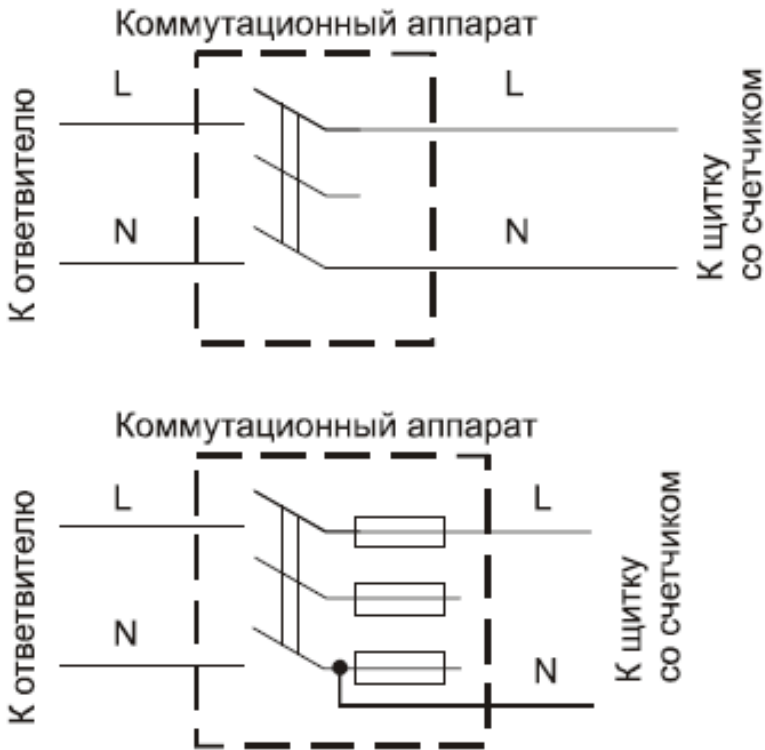
Рис. 1.16. Подключение трехполюсного коммутационного аппарата к однофазному ответвлению
