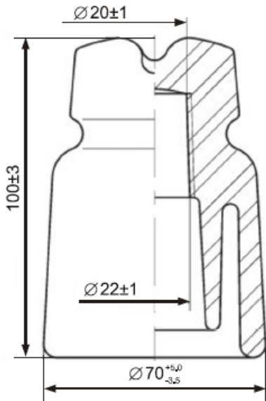
Рис. 1.6. Изолятор линейный штыревой фарфоровый типа ТФ-20 01
