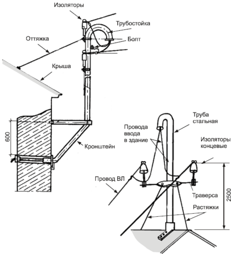
Рис. 1.14. Варианты ввода с трубостойкой
