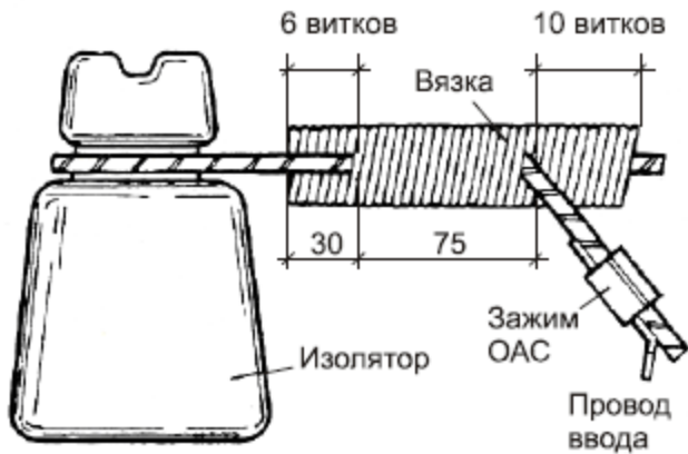
Рис. 1.12. Крепление провода ответвления к изолятору: а – зажимом; б – вязкой
