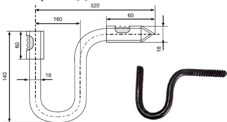
Рис. 1.9. Крюк КН-18 для крепления изоляторов ТФ-20 к деревянным опорам
