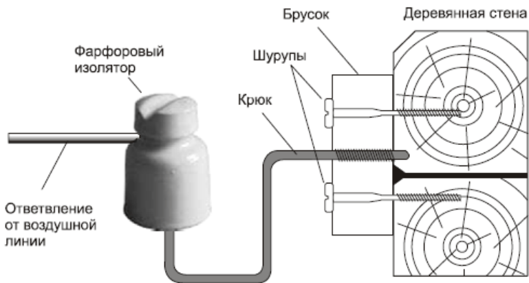
Рис. 1.10. Крепление фарфорового изолятора к стене деревянного дома
