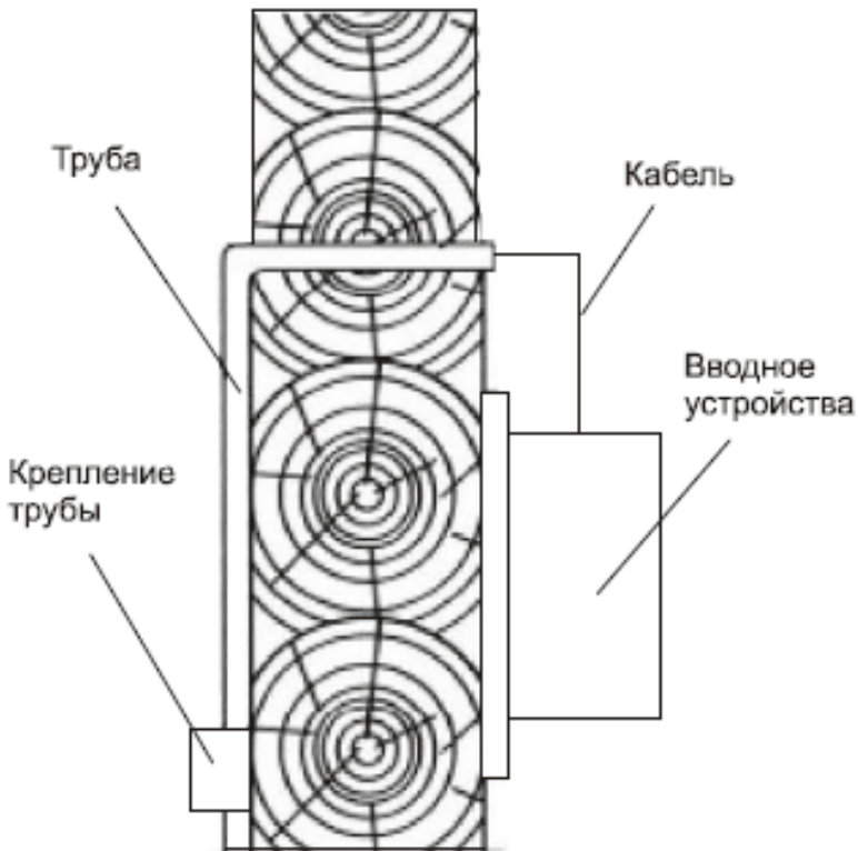
Рис. 1.5. Схема прохода кабеля сквозь стену
