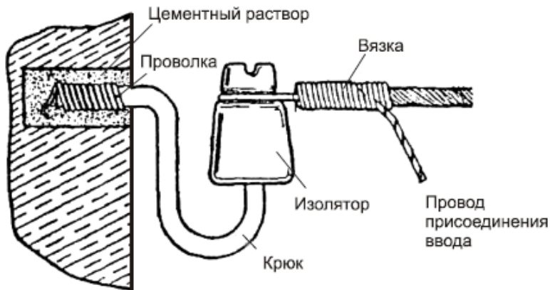
Рис. 1.11. Крепление фарфорового изолятора к бетонной стене дома
