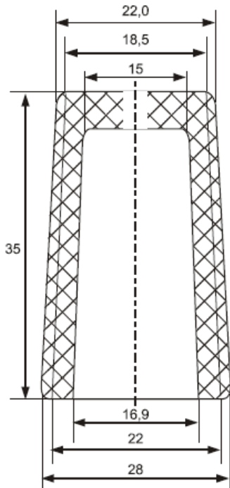
Рис. 1.7. Колпачки серии К, КП
