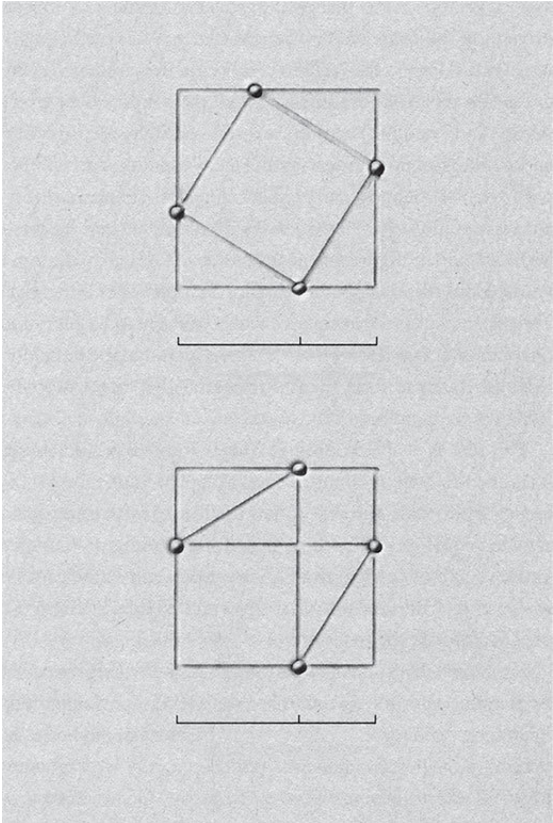
Теорема Пифагора
