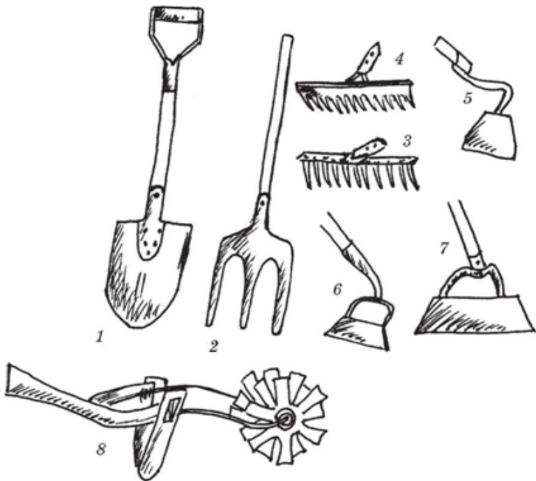
Рис. 1. Инструмент для обработки почвы: 1 – лопата для перекопки грунта; 2 – земляной бур; 3 – двойная мотыга; 4 – мотыга-рыхлитель; 5 – мотыга-грабли; 6 – широкозахватная мотыга; 7 – ступенчатая мотыга; 8 – мерка для посадки фасоли
