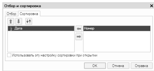
Рис. 1.8. Настройка сортировки
