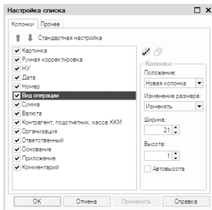
Рис. 1.9. Настройка списка
