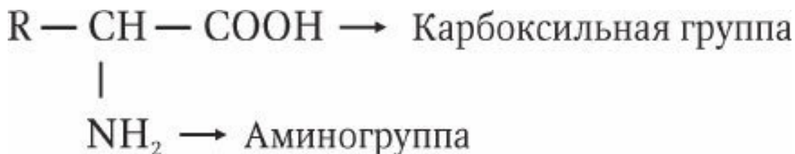
Рис. 2.1. Структура аминокислоты
