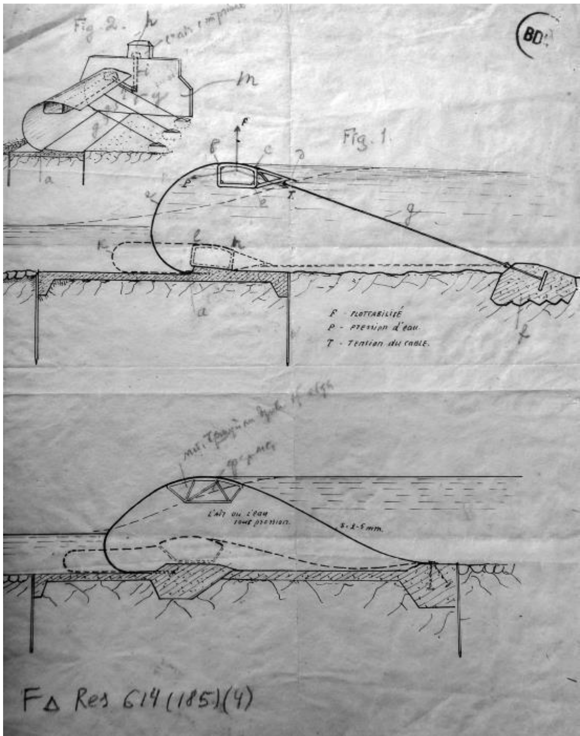
Чертеж гибкой плотины, выполненный Замятиным (предположительно начало 1910-х годов) (BDIC, Collection E. Zamiatine – F DELTA RES 614)
