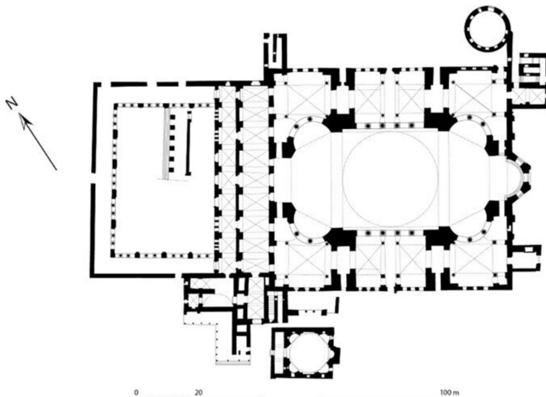
Ил. 2. План собора Святой Софии Константинопольской. Арх. Анфимий из Тралл и Исидор из Милета. 532–537 гг.
