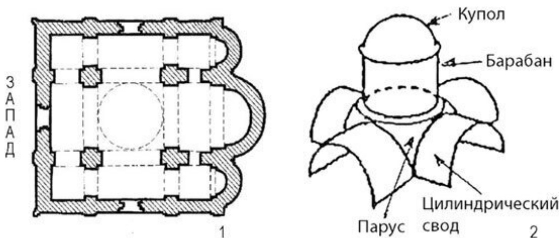
Ил. 7. Крестово-купольный храм 1. План. 2. Пространственное решение
