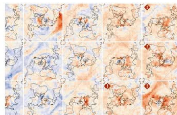
ТЕПЛОВОЙ ГРАДИЕНТ
