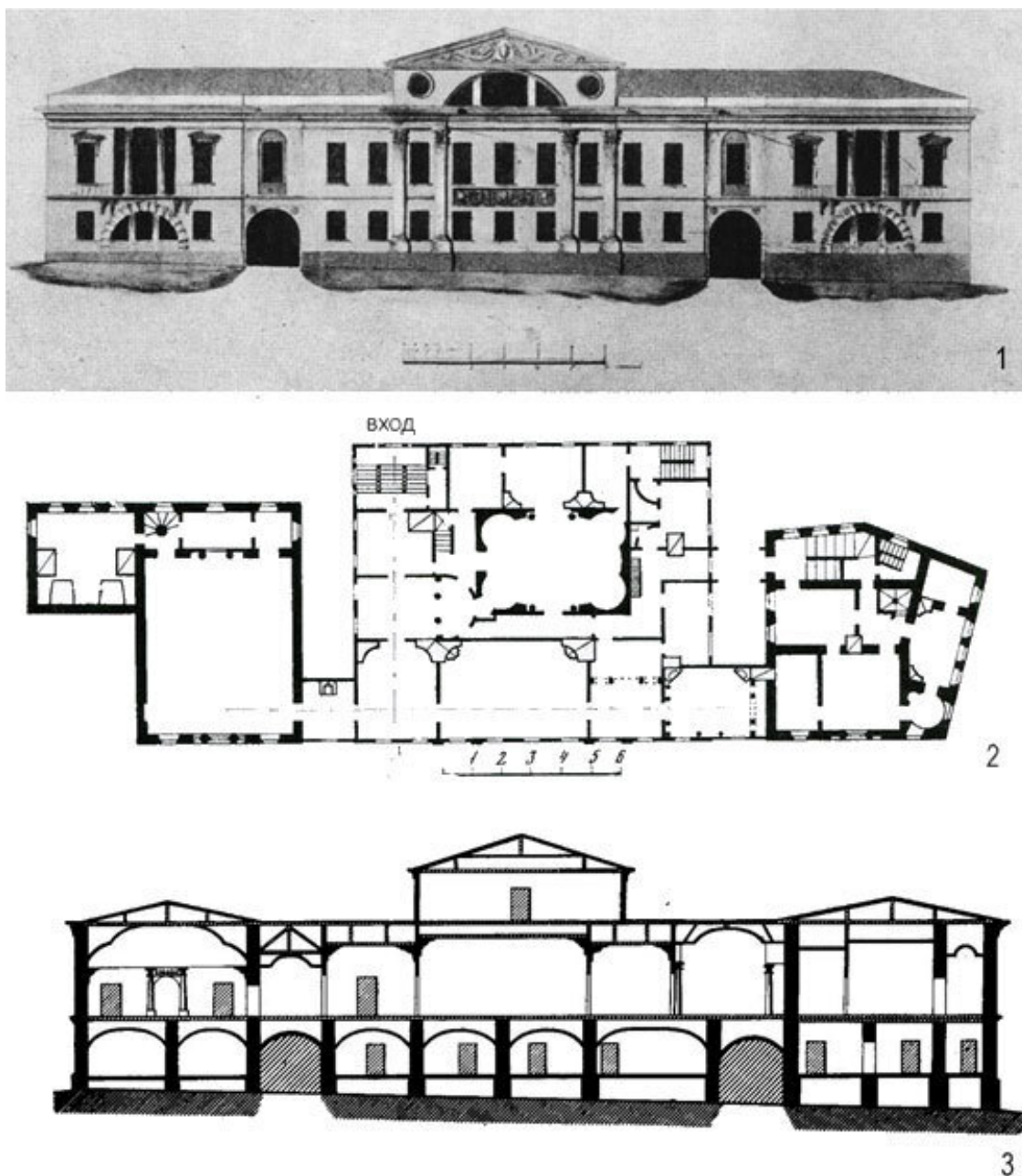
Ил. 10. Пространственный ансамбль парадных комнат. Дом Гончарова на Яузской улице в Москве. Существует на плане участка 1782 г. 1. Фасад. 2. План второго этажа. 3. Разрез
