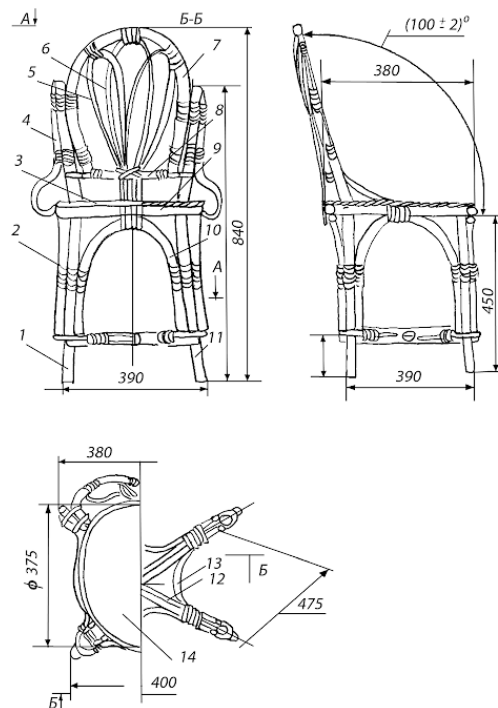
1 и 11 – ножка; 2 – кольцо сиденья; 3 – сиденье; 4 – обкладка сиденья; 5 – обмотка мест крепления; 6 – подлучка; 7 – подстрелка; 8 – обтяжка проножки; 9 – прут проножки
