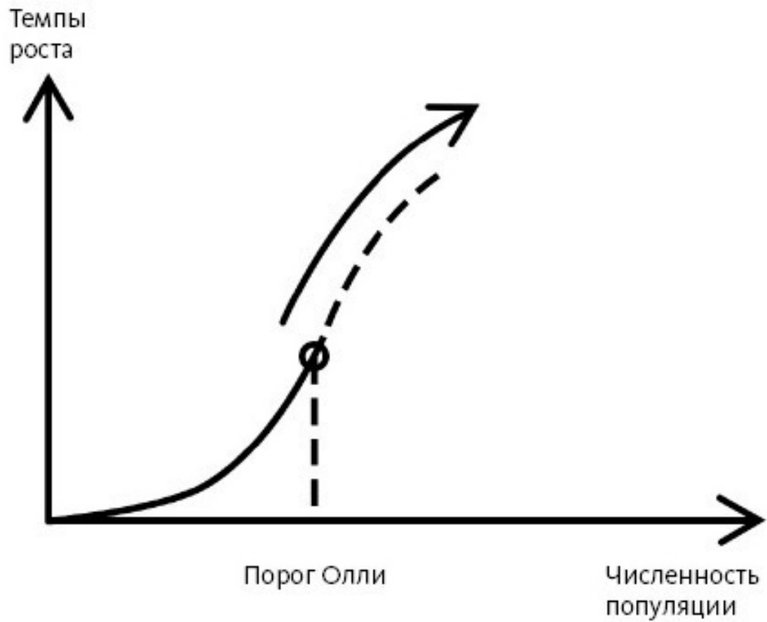
Рис. 4. Динамика численности популяции, превысившей порог Олли
