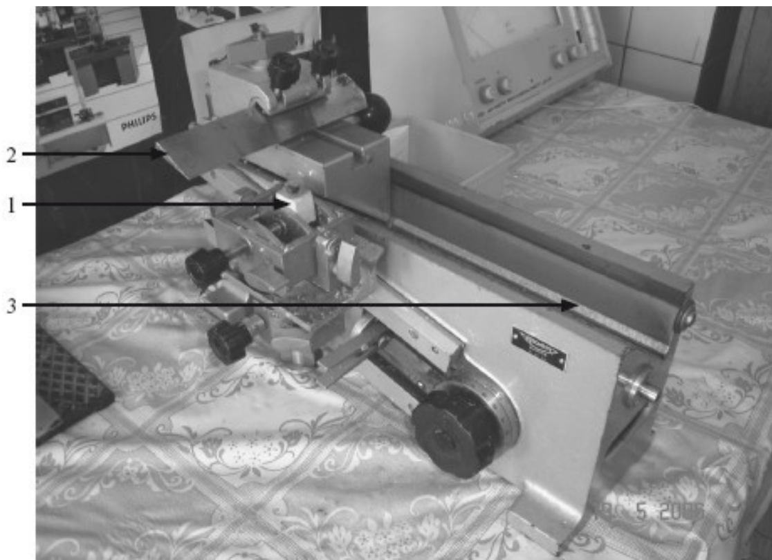
Рис. 1.1. Санний микротом.
