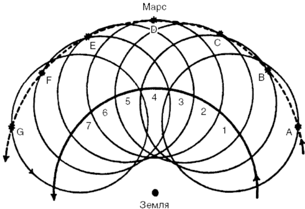
Рис. 2. Движение Марса по Птолемею 1–7 – последовательные положения центра эпицикла (тонкая линия) с интервалом в один месяц. Деферент – толстая линия. А – G – соответствующие положения планеты на эпицикле в процессе его вращения. Пунктирная линия – видимый путь планеты
